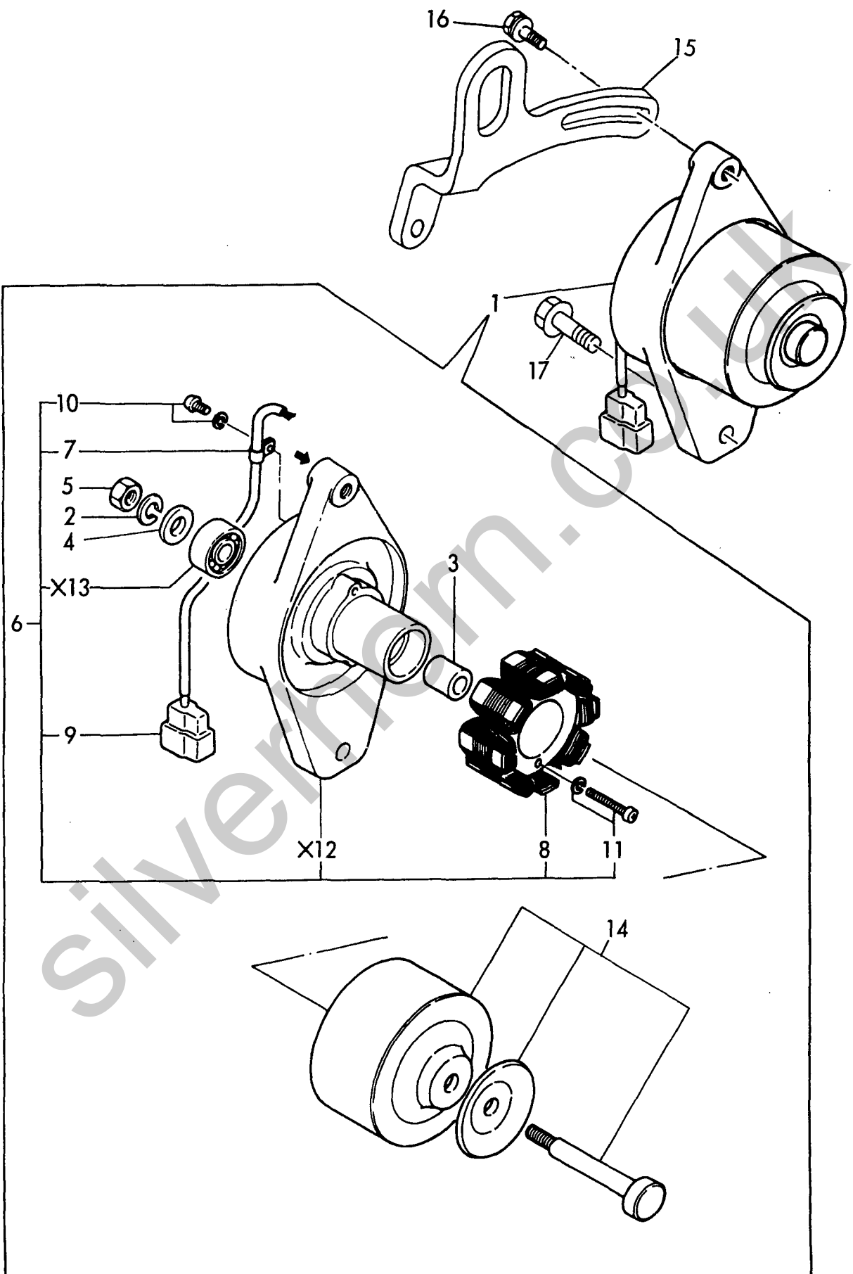
Fig. 14 GENERATOR
